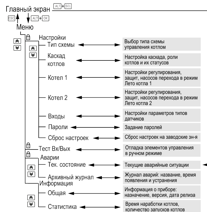
Рисунок 7.3 – Схема переходов по меню
