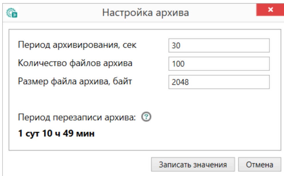
Рисунок 8.15 – Настройка архива
