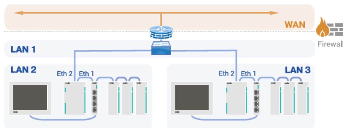
Рисунок 2.10 – Схема №3 сетевых портов контроллера ПЛК200
