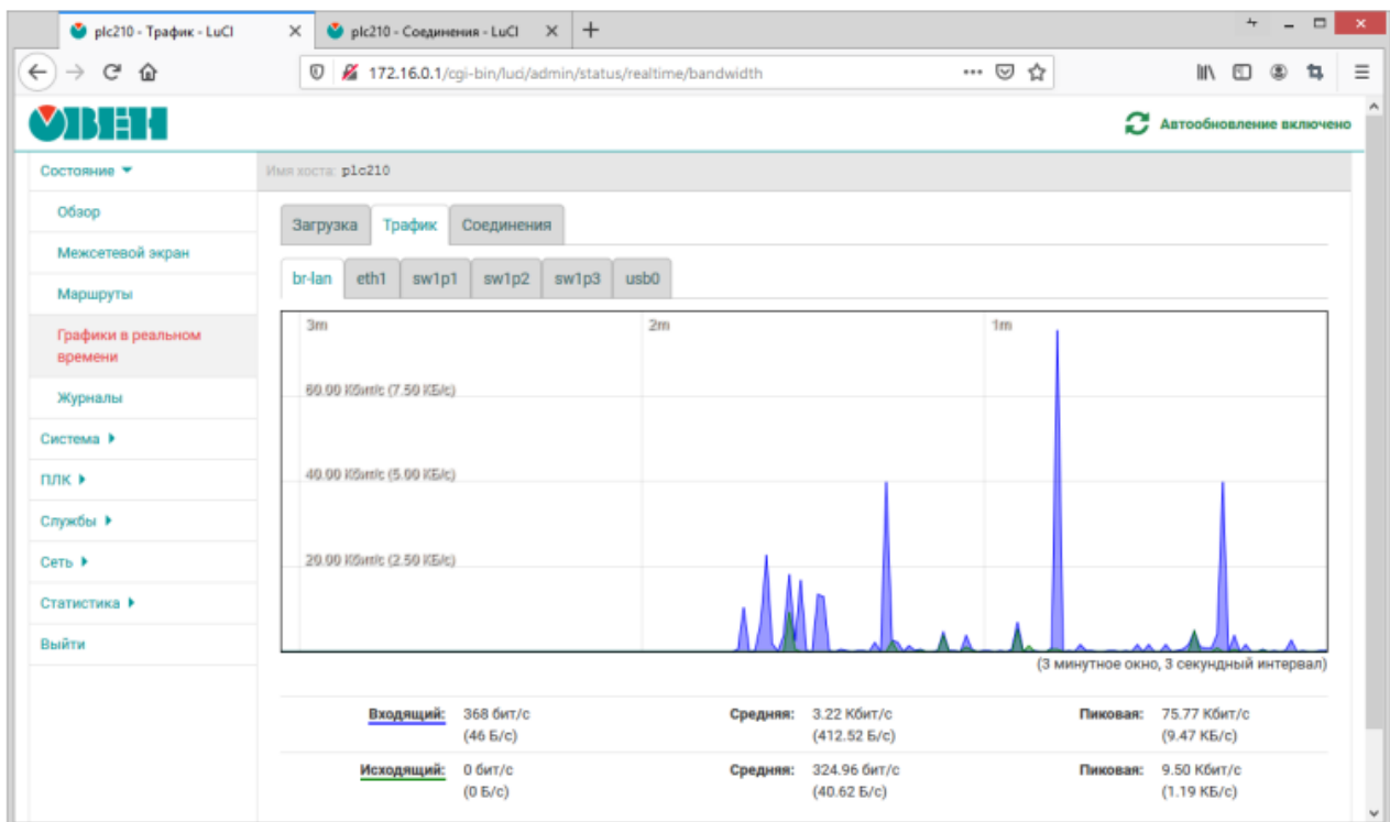
Рисунок 3.15 – Страница «Графики в реальном времени». График трафика моста «br-lan»
