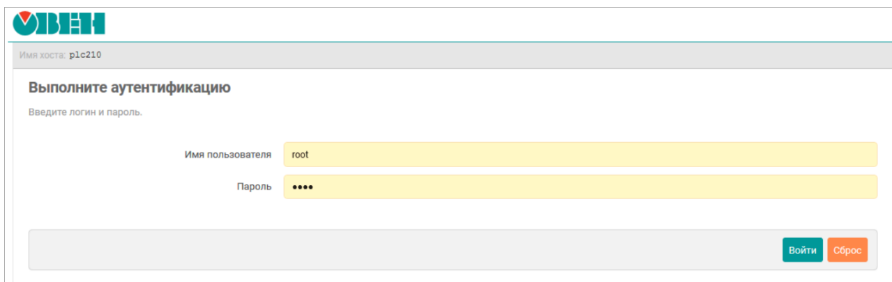
Рисунок 1.2 – Страница аутентификации
