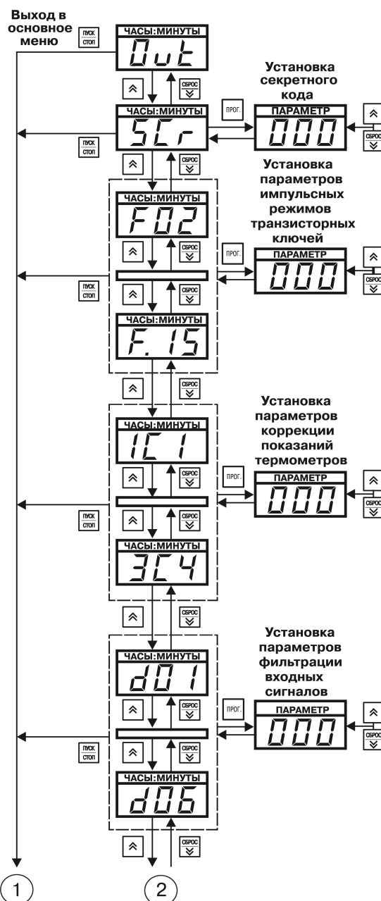
Рисунок 7.5 – Схема настройки на уровне L2 (начало)
