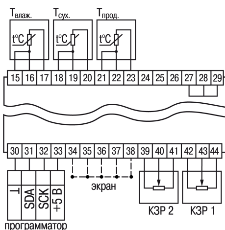
Рисунок 5.3 – Подключение измерительных датчиков и датчиков положения задвижек
