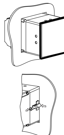
Рисунок 4.1 – Монтаж прибора
