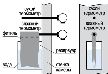
Рисунок Б.1 – Крепление датчиков температуры перпендикулярно стенке камеры
