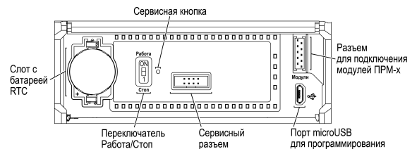
Рисунок 16 – Лицевая панель под крышкой
