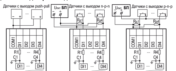
Рисунок 3 – Подключение к типу «Д»
