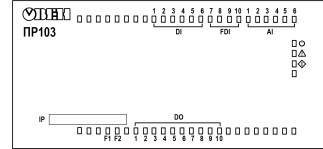
Рисунок 15 – Пример лицевой панели прибора
