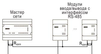
Рисунок 12 – Типовая схема подключения в режиме Master
