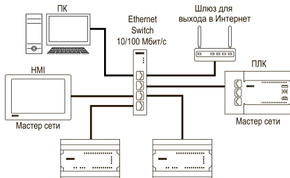
Рисунок 13 – Подключение по схеме «Звезда»
