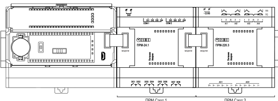
Рисунок 14 – Расположение модулей расширения на шине
