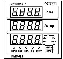
Рисунок 6.2 – Лицевая панель
