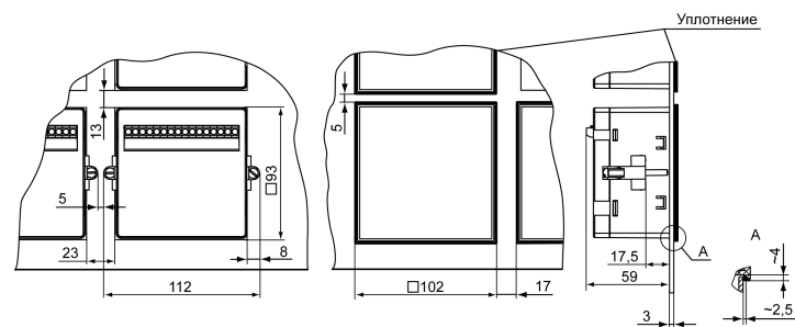
Рисунок 4.3 – Прибор в корпусе Щ1, установленный в щит толщиной 3 мм
