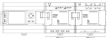
Рисунок 16 – Расположение модулей расширения на шине
