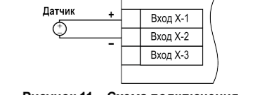
Рисунок 11 – Схема подключения активного датчика с выходом в виде напряжения 0...5 В и 0...10 В
