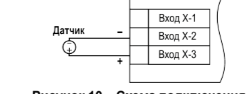
Рисунок 10 – Схема подключения активного датчика с выходом в виде напряжения -50...+50 мВ или 0...1 В
