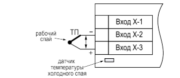
Рисунок 8 – Схема подключения термопары
