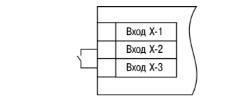
Рисунок 6 – Схема подключения к дискретному входу
