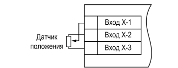
Рисунок 7 – Подключение датчика положения резистивного типа
